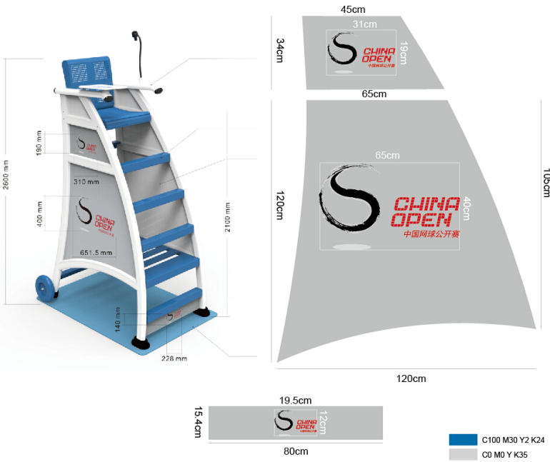
主裁座椅尺寸标注
